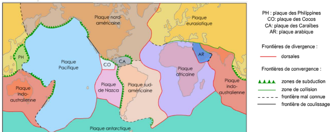
Carte des 12 plaques tectoniques identifiées à la surface du globe
